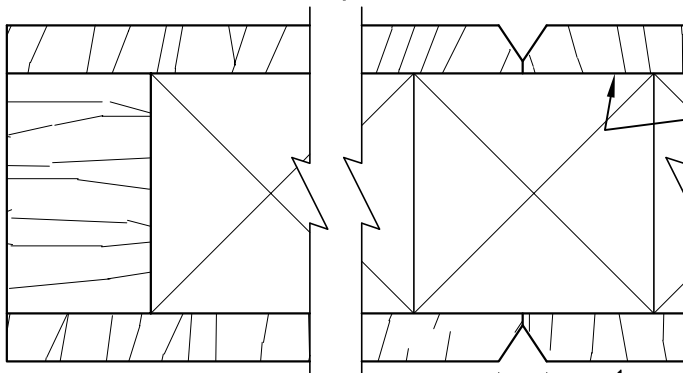
LVD STANDARD PLANK DOOR V Grooves Optional
